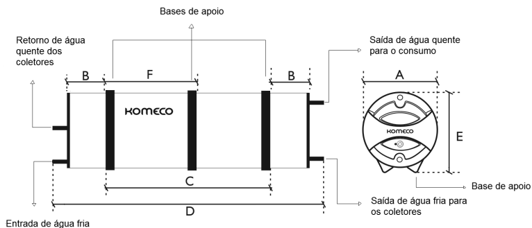
Ficha Técnica dos Reservatórios Térmicos Komeco
